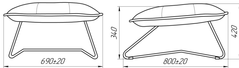
Рисунок 4 – М1965-18 (банкетка)
