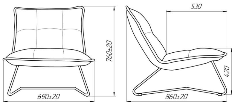
Рисунок 1 – М1965 (стул)
