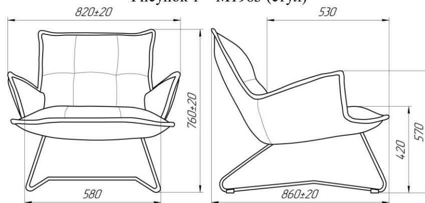
Рисунок 1 – М1965 (стул)
