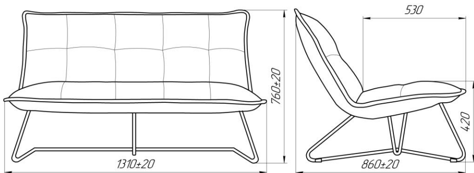
Рисунок 3 – М1965-22 (диван)
